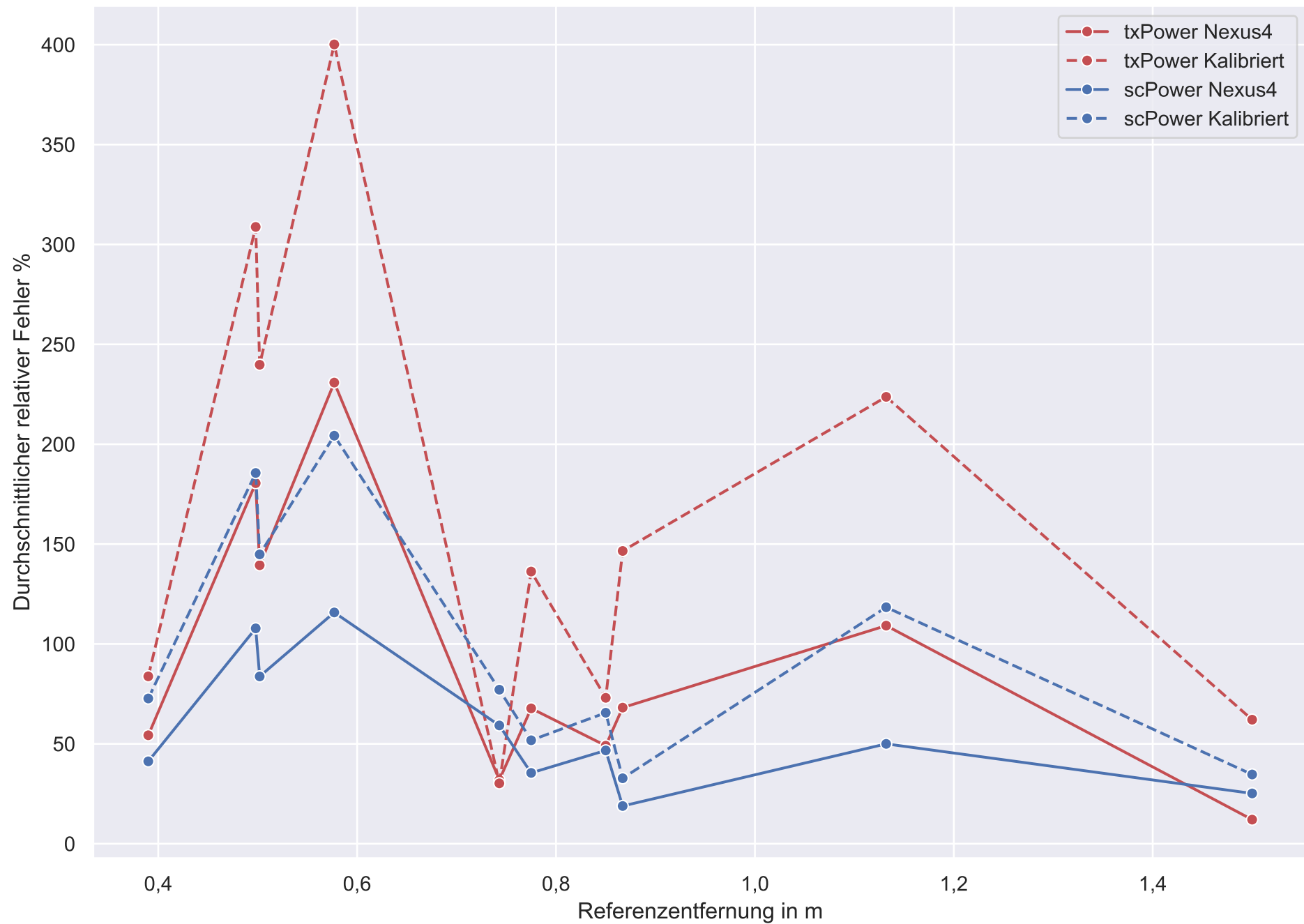
Fehler bei der Distanzberechnung mit und ohne Kalibrierung
